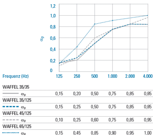
Schallabsorptionsgrad α p , pinta WAFFEL Material willtec, nach DIN EN ISO 11654
