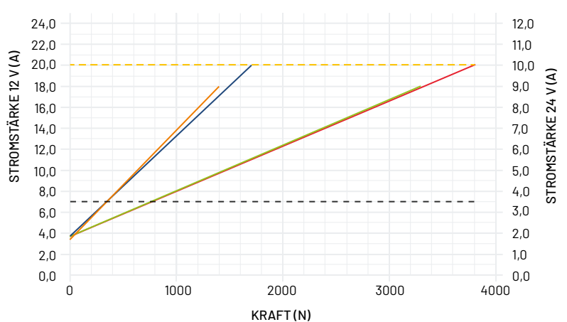
Positioniersystem – Verhältnis Kraft/Stromstärke
